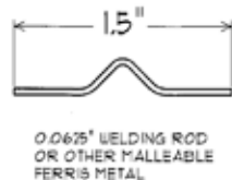
(D) WIRE RETAINER
